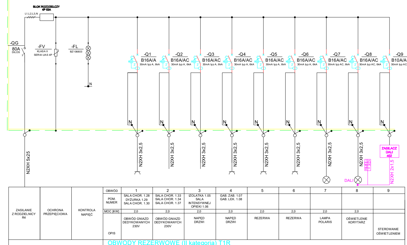
OBWODY REZERWOWE (III kategoria) T1R
