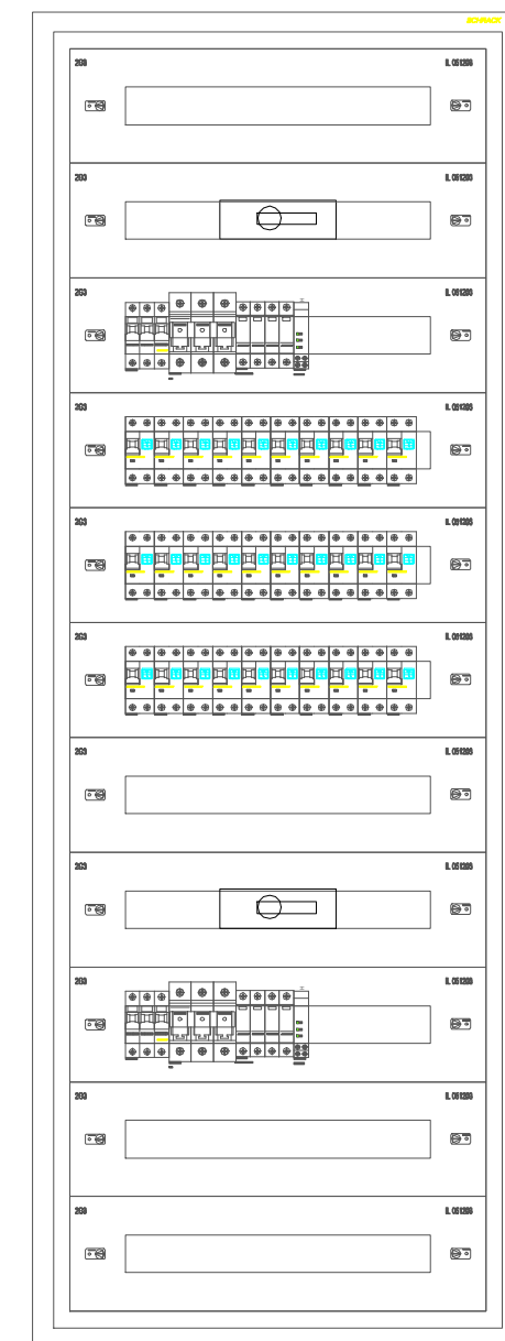
Obudowa podtynkowa 1605x590x250
