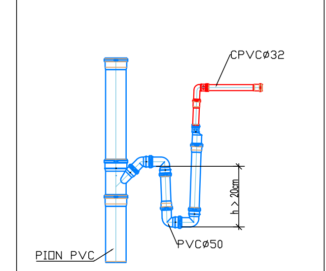
SZCZEGÓŁ WŁĄCZANIA INSTALACJI ODPROWADZANIA SKROPLIN DO INSTALACJI KANALIZACYJNEJ
