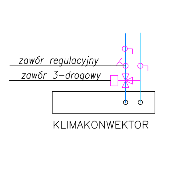
SCHEMAT PODŁĄCZENIA KLIMAKONWEKTORA-CHŁODZENIE
